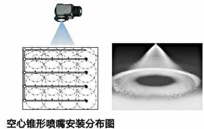
空心锥形喷嘴安装分布图
