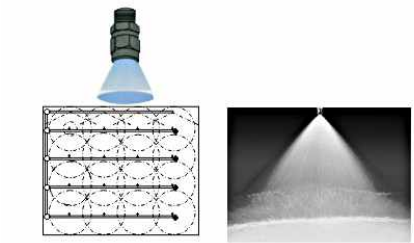
实心锥形喷嘴安装分布图
